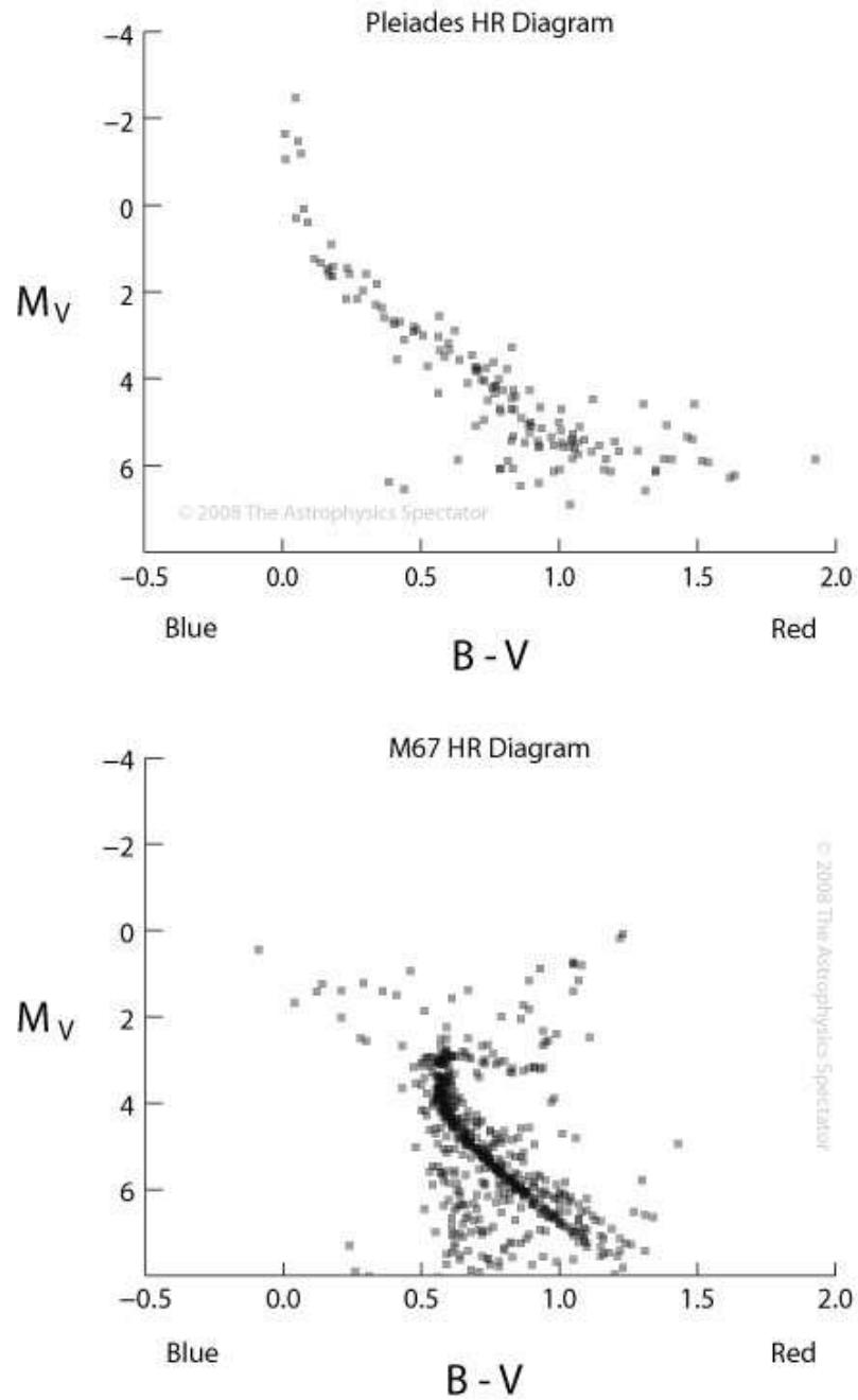
Figur 1: Hertzsprung–Russell-diagram for to åpne (galaktiske) stjernehoper, Pleiadene (Sju-stjernen) og M67 (nr. 67 i Messiers katalog). Horisontalaksen viser fargeindeksen B - V , vertikalaksen viser den absolutte størrelsesklassen (magnituden) M_V målt med et V-filter som slipper gjennom synlig lys. Figurene er tegnet av Jerome James Brainerd.
