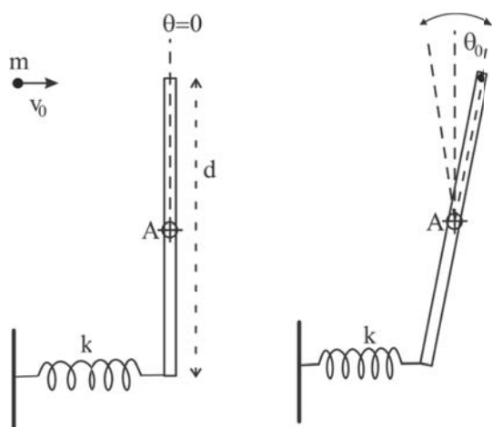
Figur 2 Skjematisk skisse av vertikal stang opplagret i aksene A gjennom midtpunktet.
