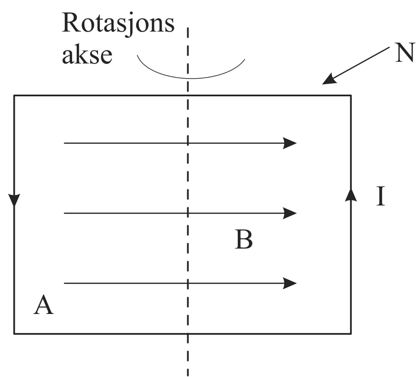
Figur. Spole med N viklinger i magnetfelt.
