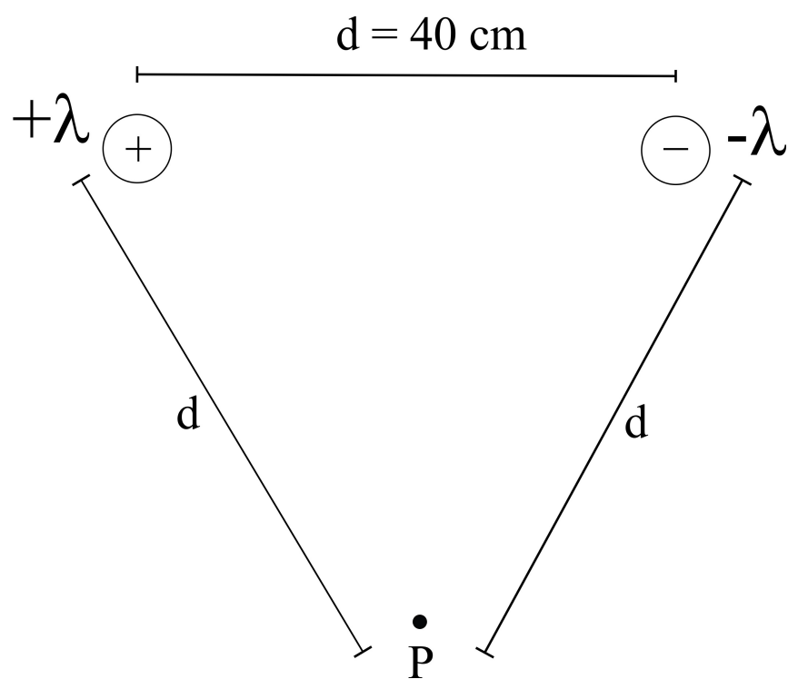
Figur. Illustrasjon av to svært lange, lineære og parallelle ledere med motsatt ladningstettleik og et punkt P. Innbyrdes avstander mellom lederne er d , og avstand fra P til hver av lederne er d . Illustrasjonen viser et tverrsnitt i planet kor punktet P e. Lederne står normalt på planet i figuren.
