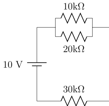
Figur 6: En resistiv krets
