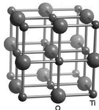
III - TiO
