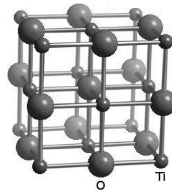
III - TiO
