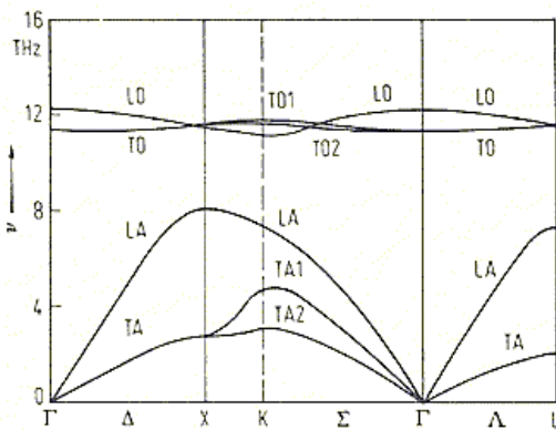
Fonon dispersjonsrelasjonsrelasjon
