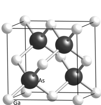
I - GaAs
