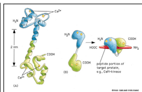
Calmodulin
