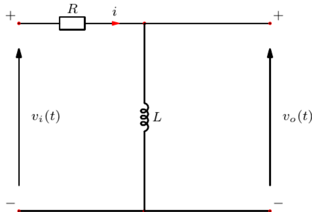
Figur 5: Høypassfilter; spørsmål 4
