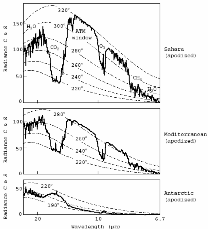
Figur 1. Spektrale målinger av jord/atmosfære system målt med et spektrometriometer i nadir posisjon plassert på satellitt i polar bane.
