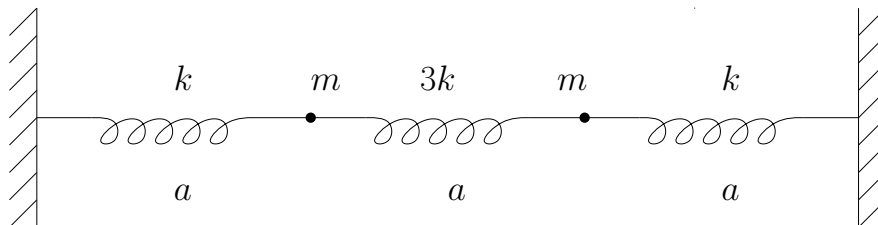
Figur 5: Massane og fjørene i systemet under betraktning i Oppgåve 3b.
